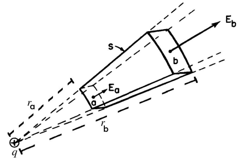
Figura 2.5: Superfície Gaussiana com dois segmentos esféricos. (Feynman)
